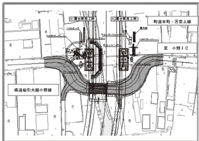
小野橋架け替え工事(迂回路)
